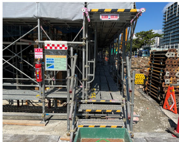
写真② 仮設通路段差・突出部へのトラテープ表示例
