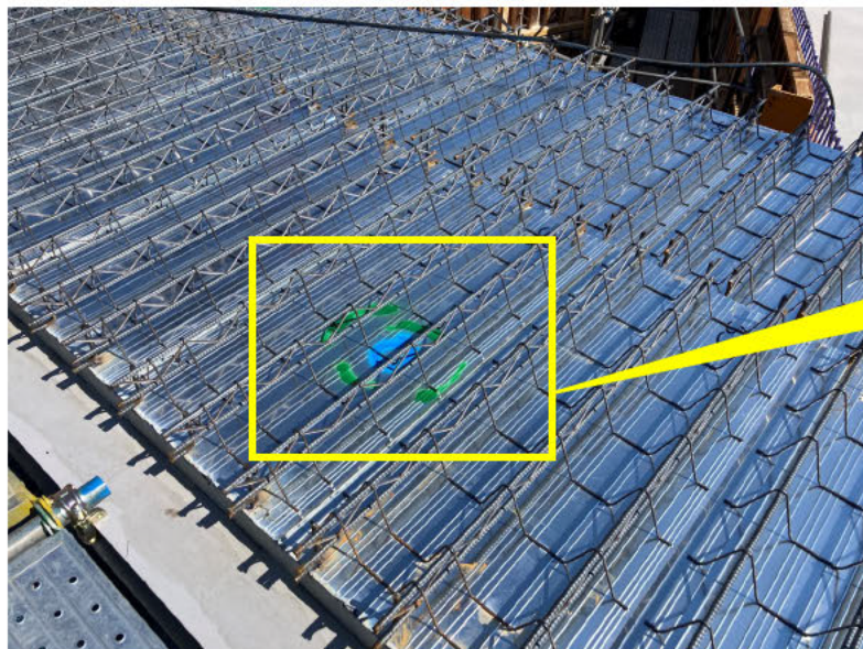
写真① デッキスラブへの固定完了表示
