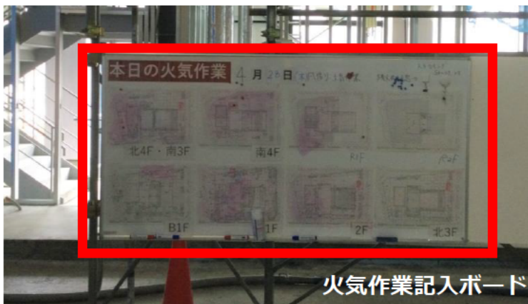
各階の平図面に火気作業場所を作業員が記入する
