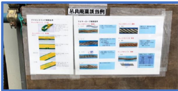
玉掛けワイヤー、スリングベルトの 廃棄基準を示した写真
