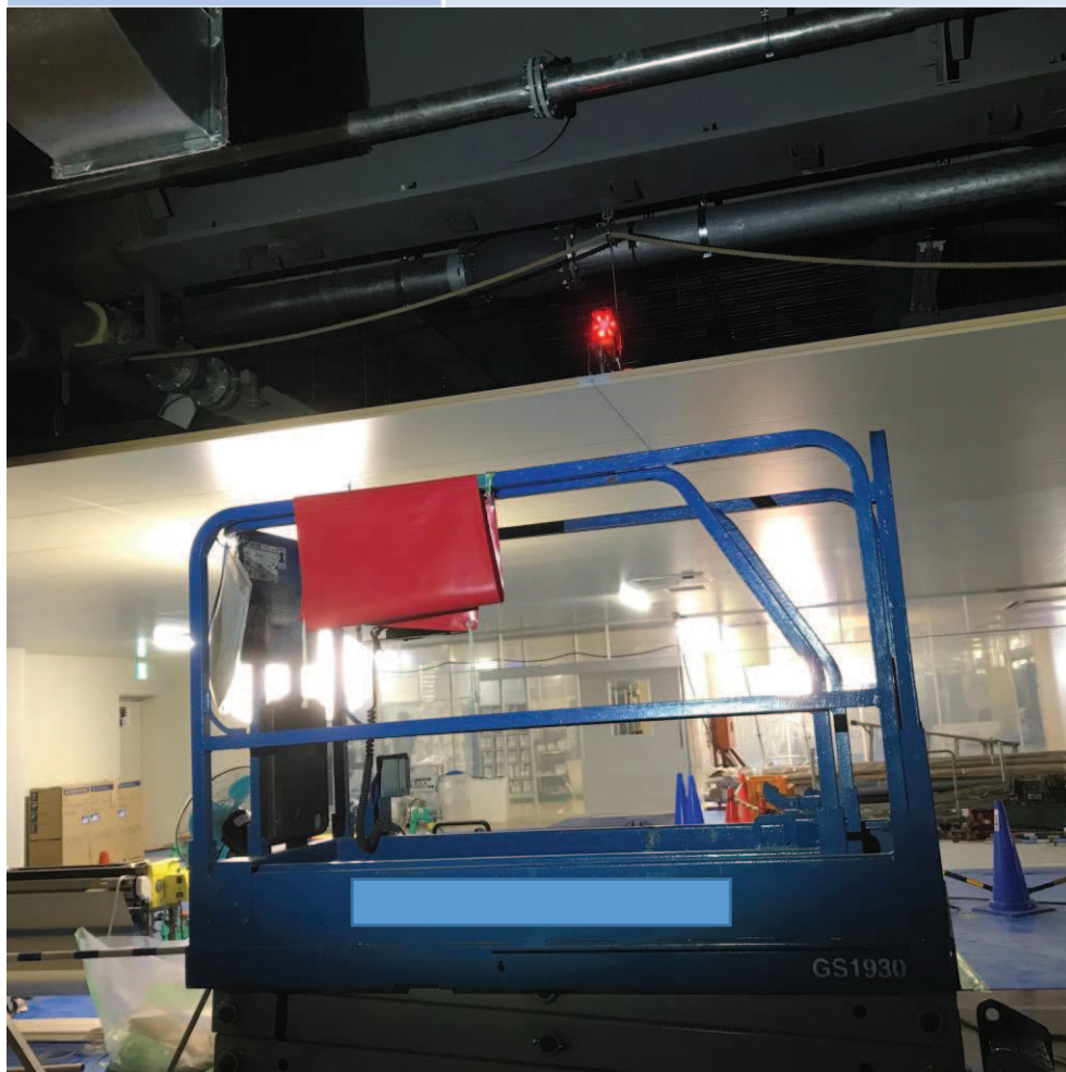
天井端部写真
