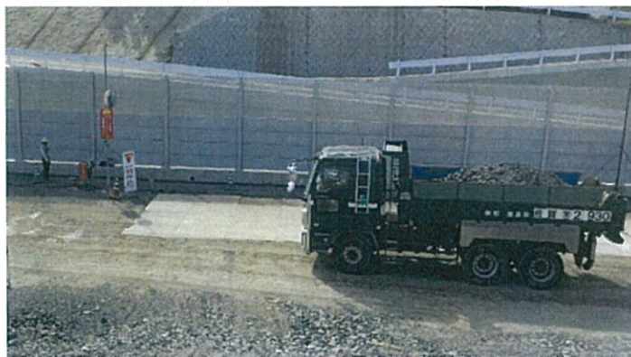
出入り口手前に設置した「ダンプ荷台とクレーンブーム用ミラー」を使用して荷台積載状況とブームの格納忘れを確認して場外へ
