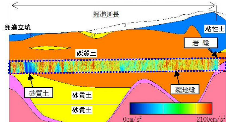
地質実績図 (コンター表示)
