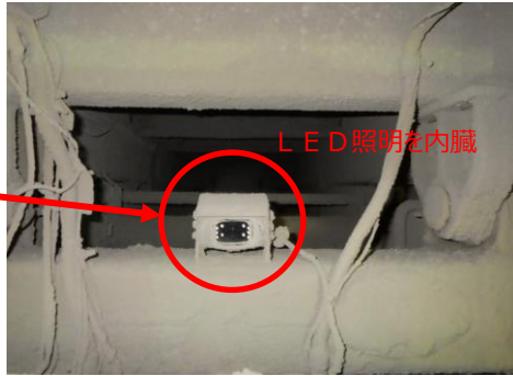
LED照明内臓バックカメラ ダンプトラック取付け状況
