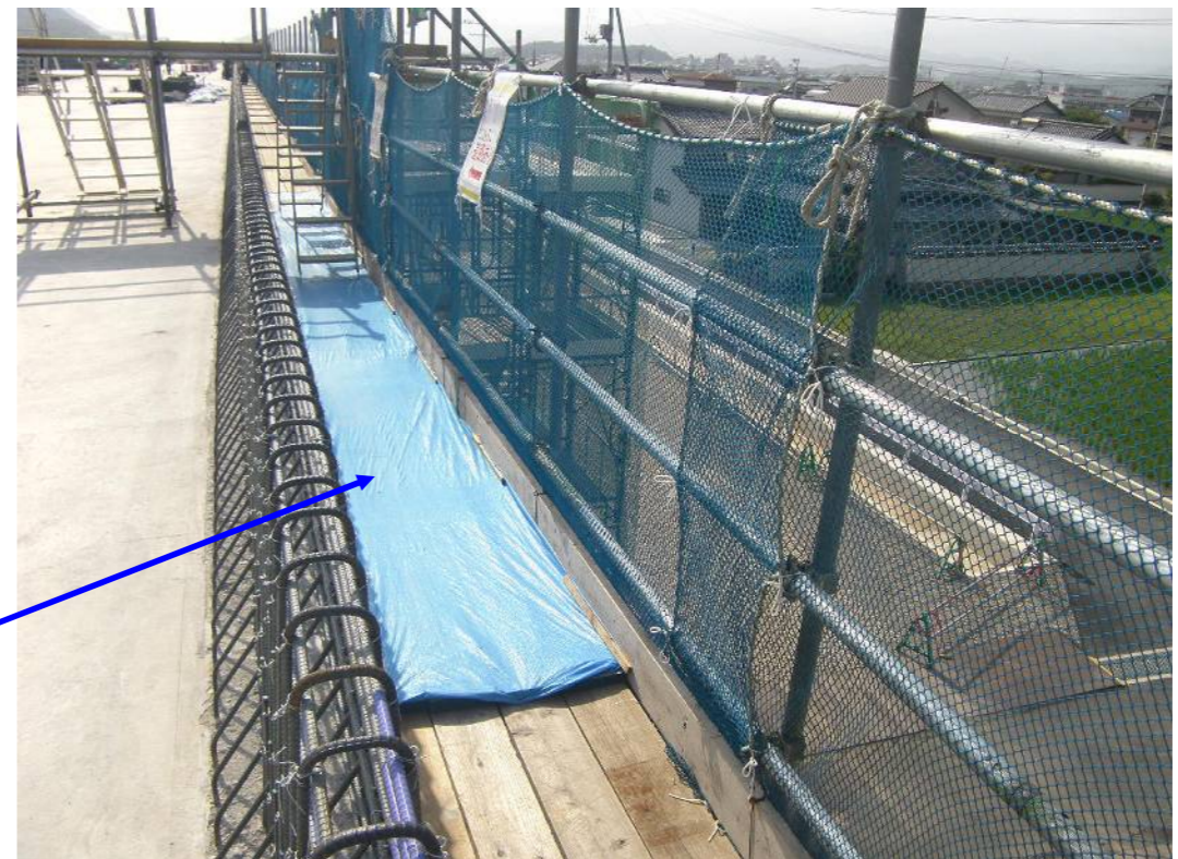
③張出足場上はシート養生
