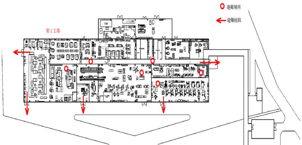
神岡セラミック 第1・第2工場 震災時緊急避難場所・避難経路図（夏期）
