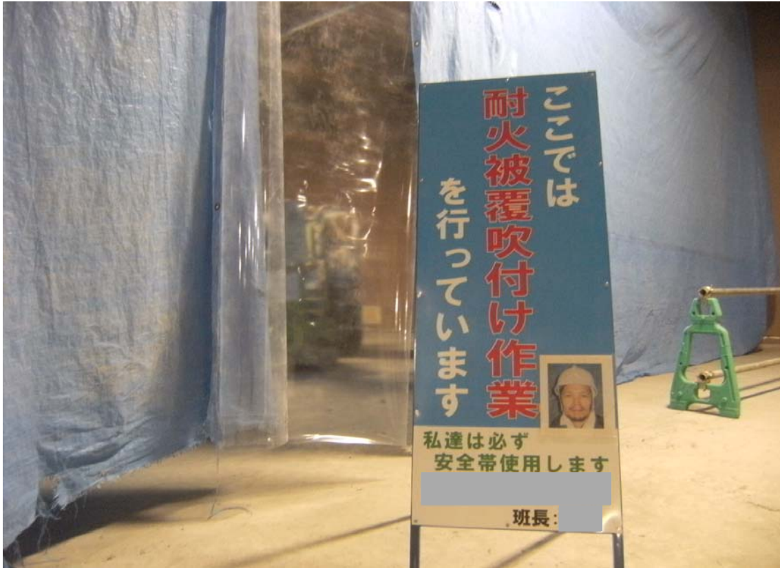
養生で作業状況がわかりにくかったため、透明フィルムにて見える化を行い、さらに作業担当者を写真付きで看板に表示して危機意識を高めさせるようにした
