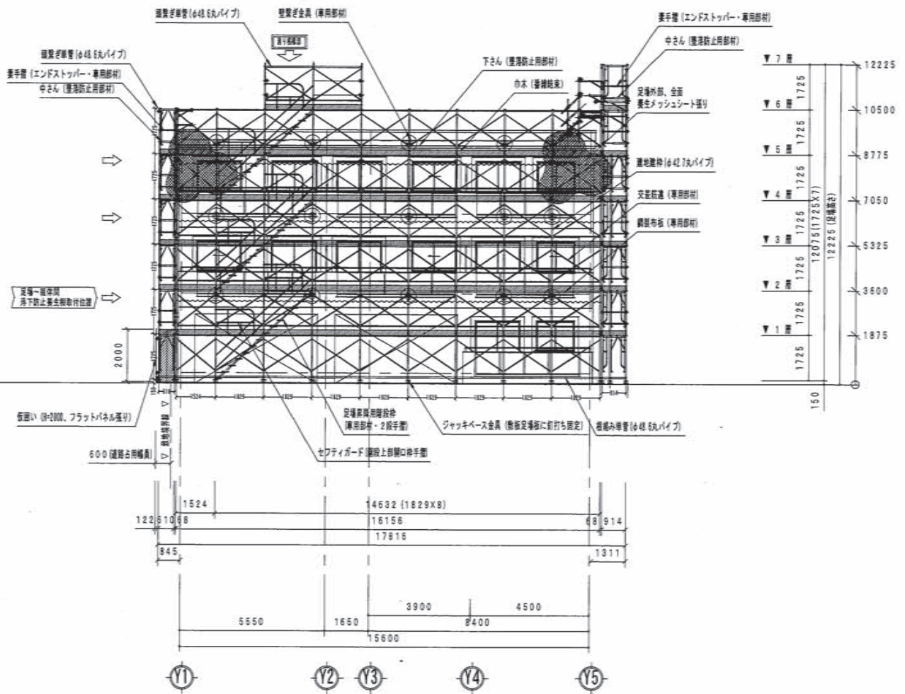
南立面図 S=1/100
